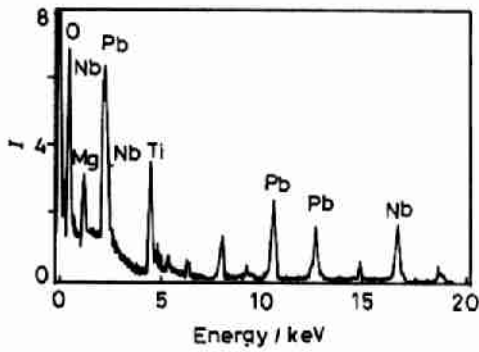
图 4 图 3 中孪生畴区的原位 EDS 谱
