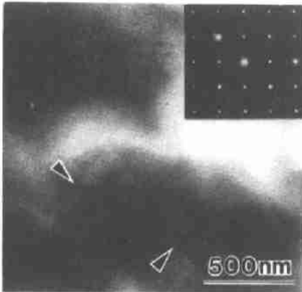
图 6 透明单晶 (001) 晶片中畴结构典型的 TEM 像及选区电子衍射斑点
