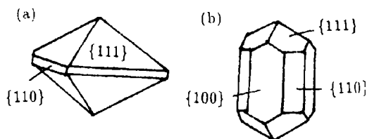
图 6 锆石晶体的结晶形貌
