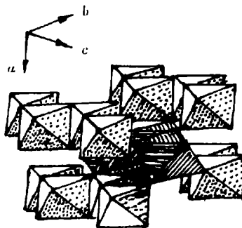
图 4 黑钨矿晶体中 [WO 6 ] 2- 八面体与 Fe 2+ -O 6 (Mn 2+ -O 6 ) 八面体的结晶方位
