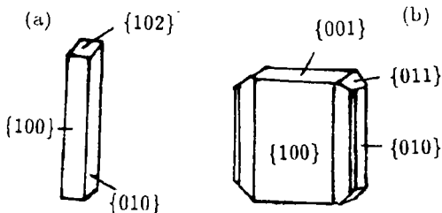
图 3 黑钨矿晶体的结晶形貌
