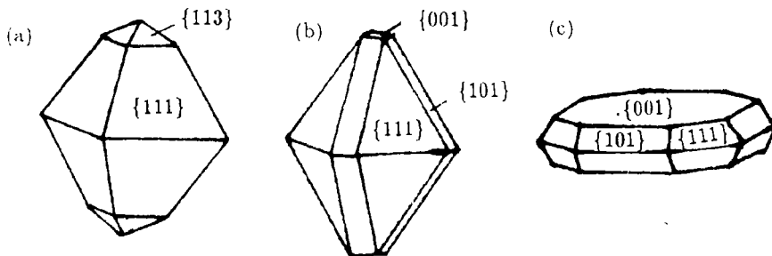
图 1 白钨矿晶体的结晶形貌 Fig. 1 Morphology of scheelite crystals
